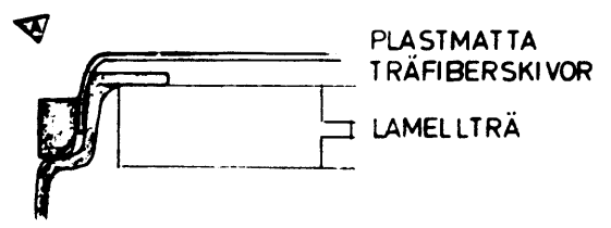
KANTSEKTION VID BRUNN
